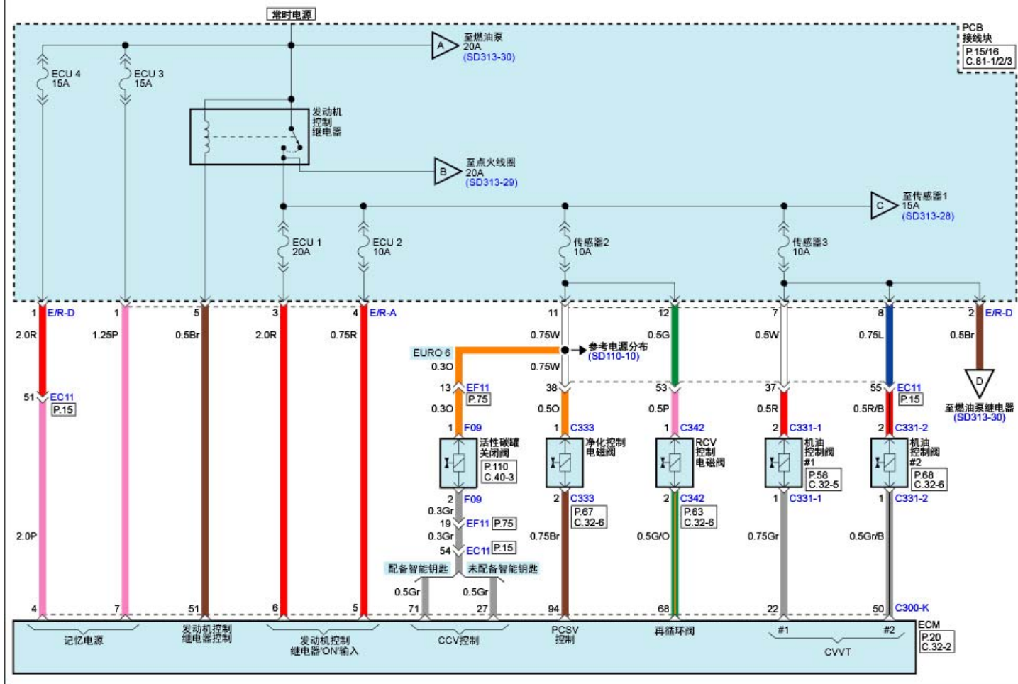
发动机控制系统(G4LD:KAPPA 1.4L T-GDI)(3)
